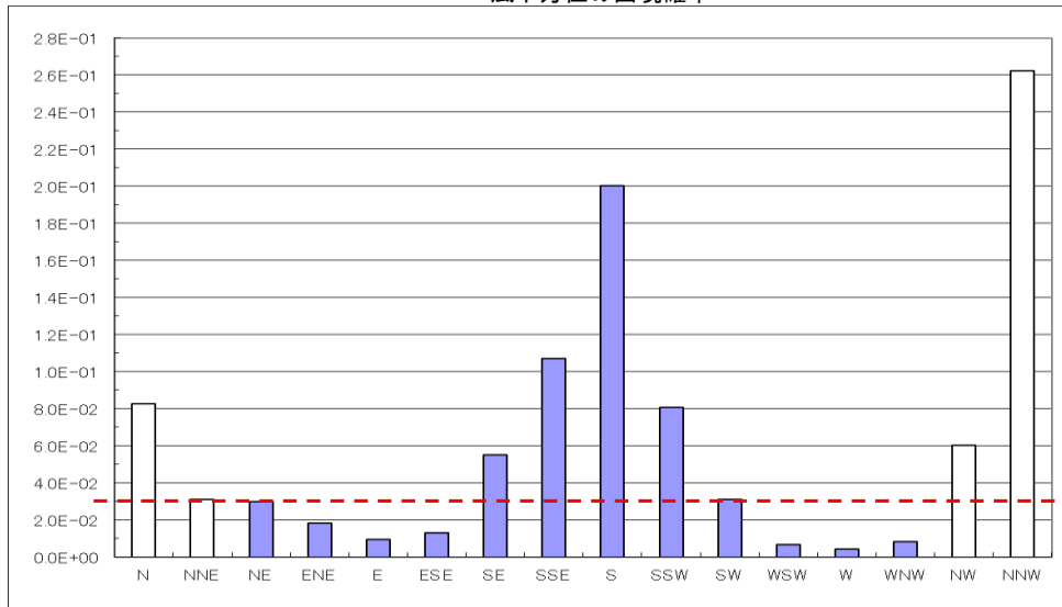
風下方位の出現確率
