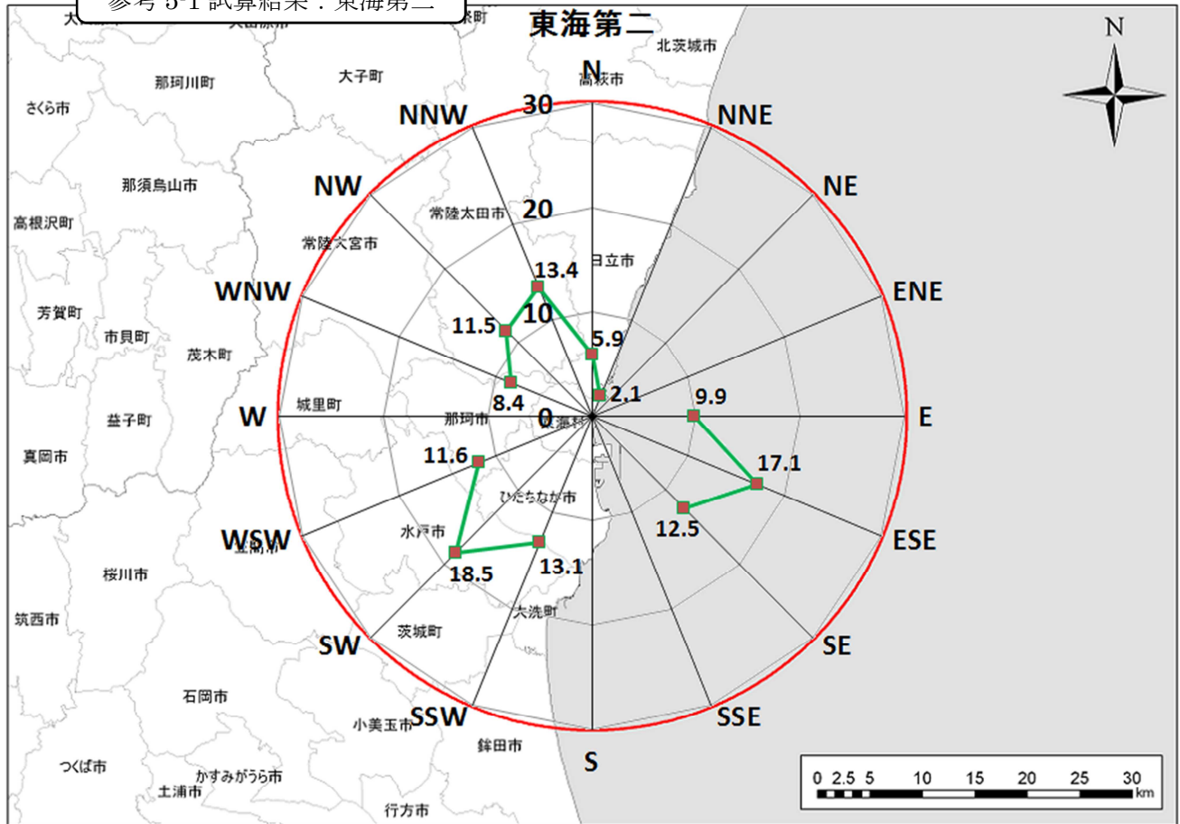
参考 5-1 試算結果：東海第二
