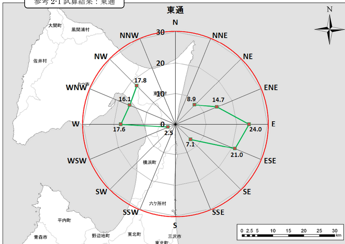
参考 2-1 試算結果：東通
