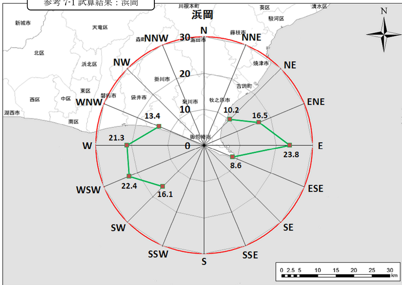
参考 7-1 試算結果：浜岡
