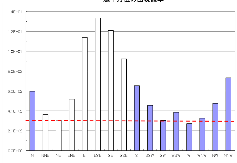
風下方位の出現確率
