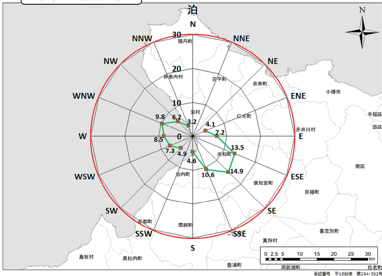
参考 1-1 試算結果：泊
