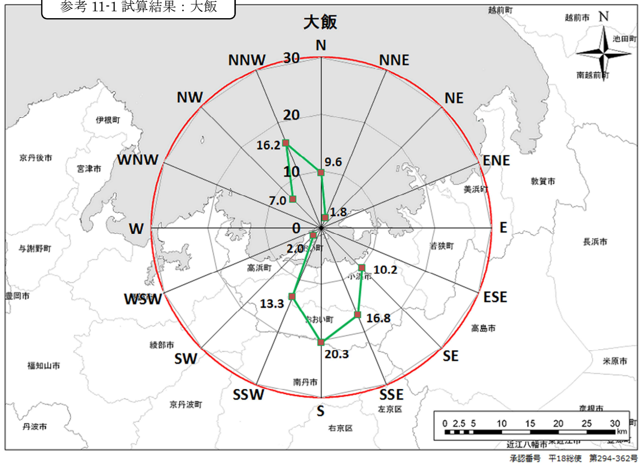
参考 11-1 試算結果：大飯
