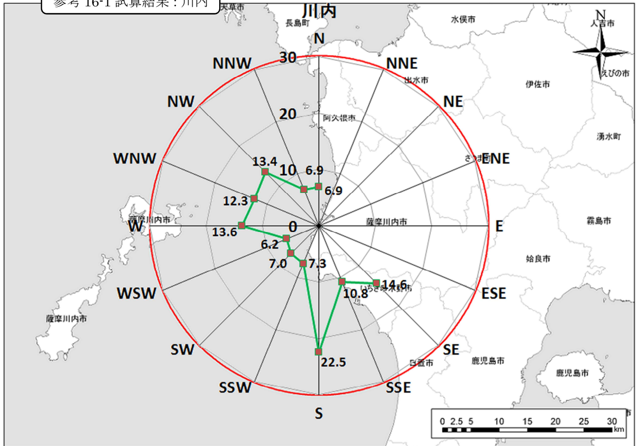
参考 16-1 試算結果：川内
