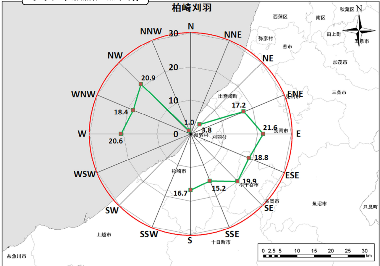
参考 6-1 試算結果：柏崎刈羽
